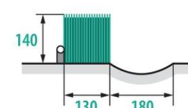
14 WAŁ Z ŻYWOPŁOTEM BANK WITH HEDGE
