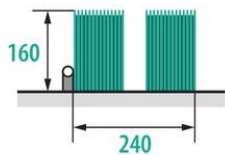
9 PRZEJŚCIE DROGI / ROAD CROSSING
