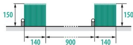
9 PRZEJŚCIE DROGI / ROAD CROSSING
