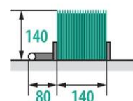
18 TUJE BRUSH FENCE
