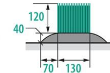
14 WAŁ Z ŻYWOPŁOTEM BANK WITH HEDGE
